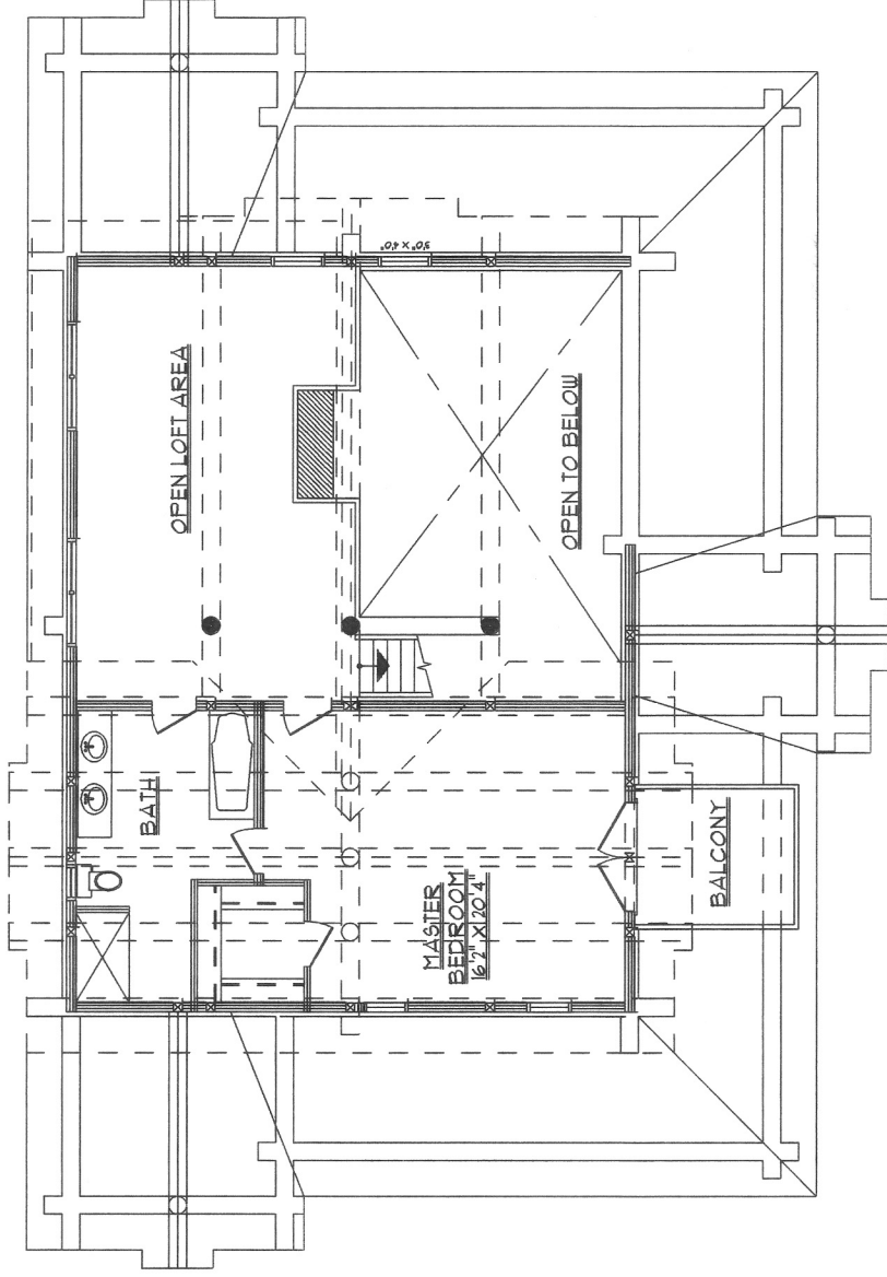
LOFT FLOOR PLAN 210 SE
